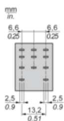
Vista laterale contatto
