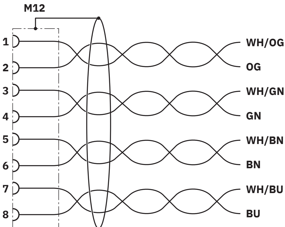
Diagrama eléctrico
