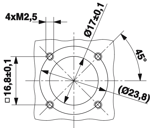
Maßzeichnung
