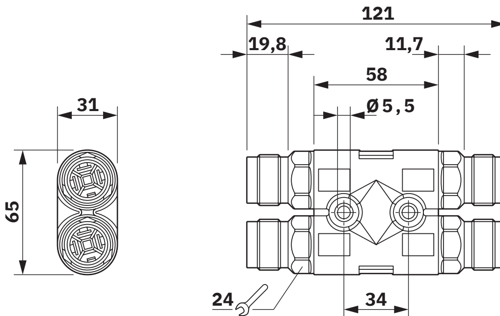
Maßzeichnung
