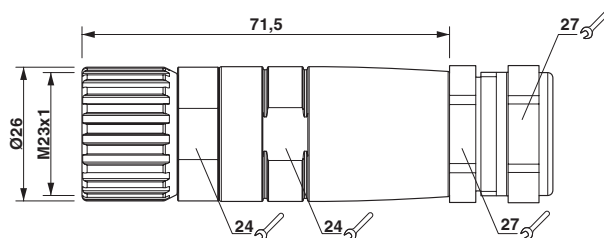
Esquema de dimensiones
