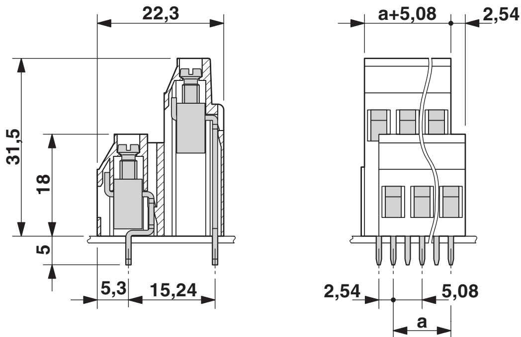
Maßzeichnung
