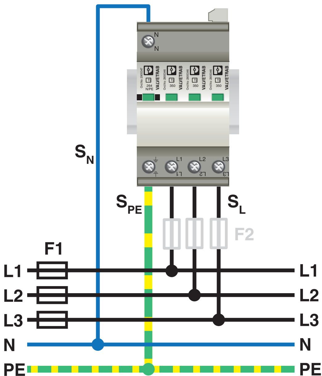
Applikationszeichnung
