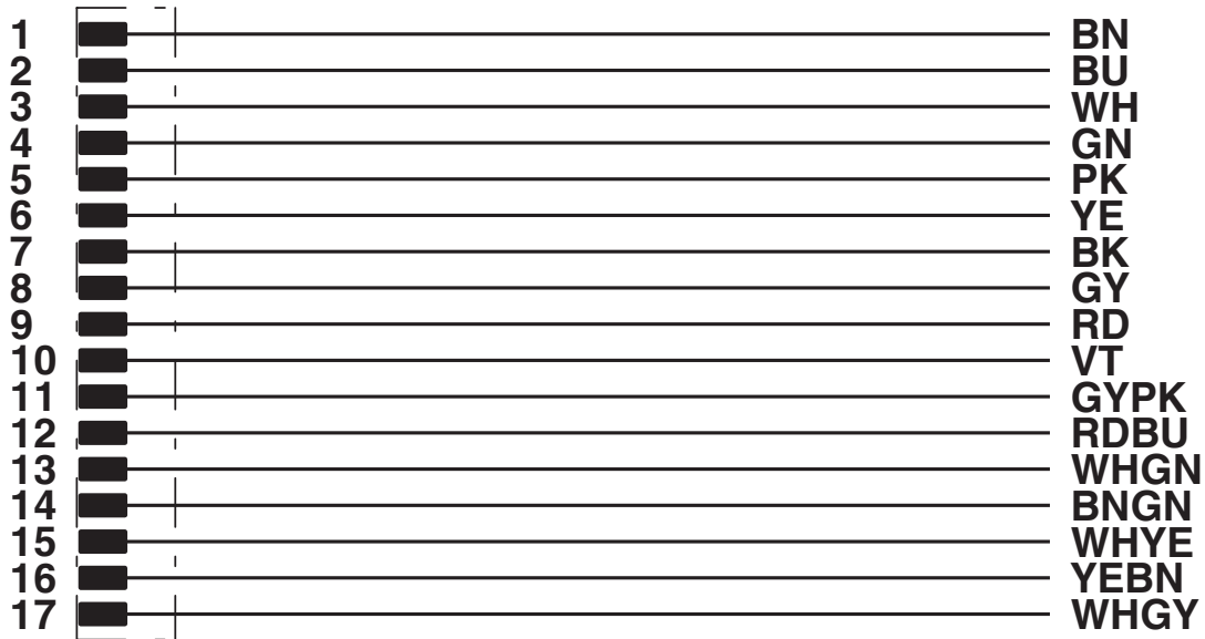
Diagrama eléctrico
