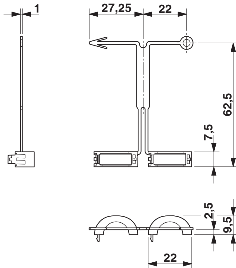
Maßzeichnung
