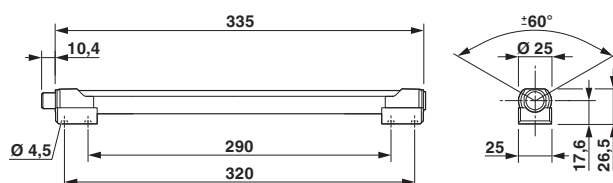
Esquema de dimensiones
