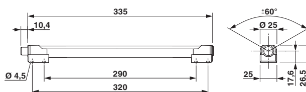
Dessin coté
