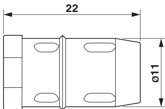
Esquema de dimensiones
