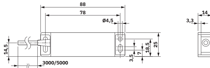
Dessin coté
