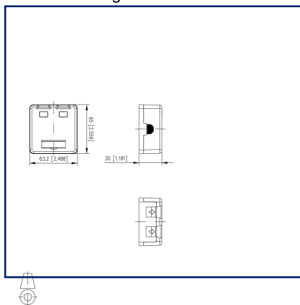
Maßzeichnung
