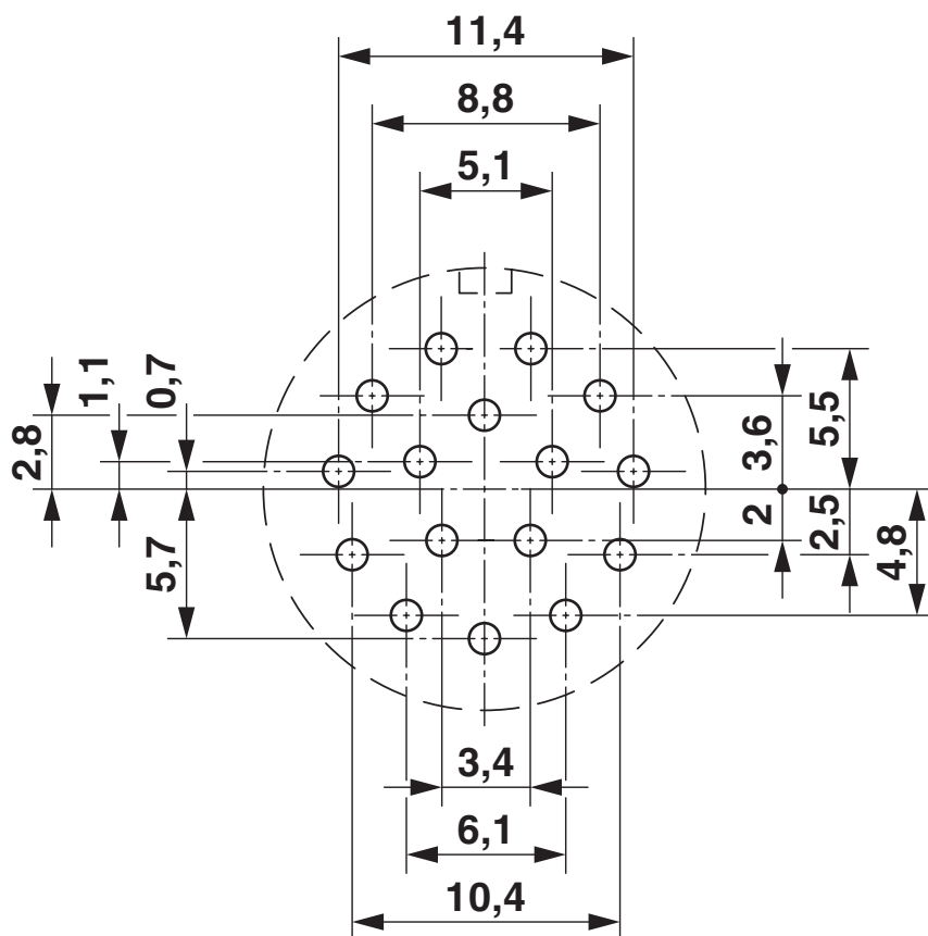
Esquema de taladros/geometría pads soldadura
