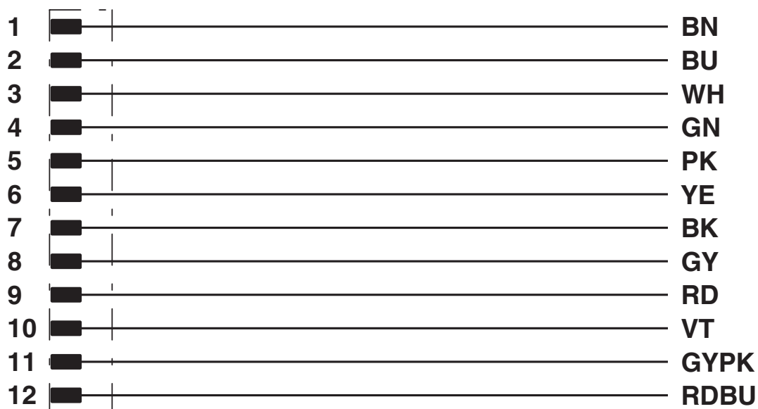
Ocupación de contactos del conector macho M12
