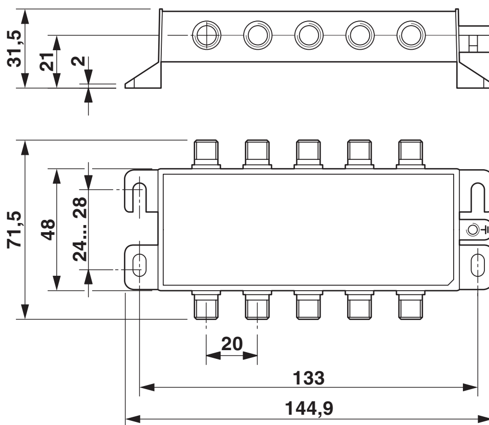
Dessin coté
