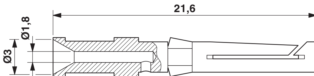
Dessin coté
