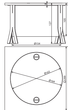
Maßbild UFTSK 200X200X105 V2A
