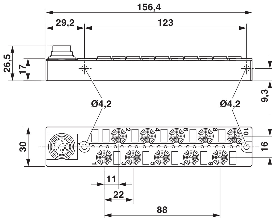
Dessin coté
