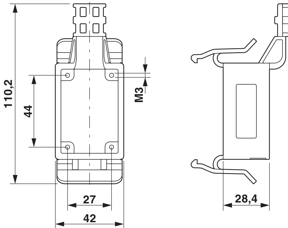
Maßzeichnung
