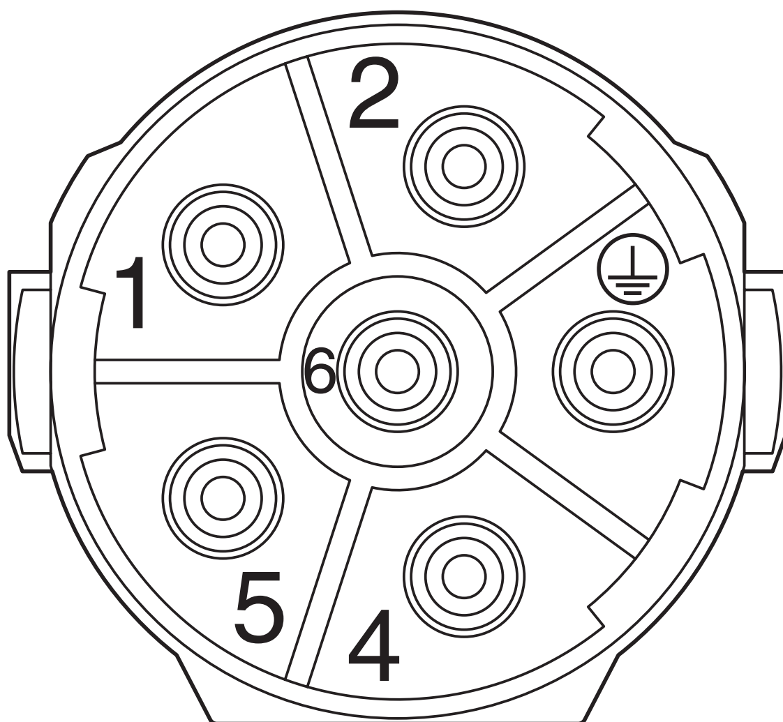
Plano esquemático
