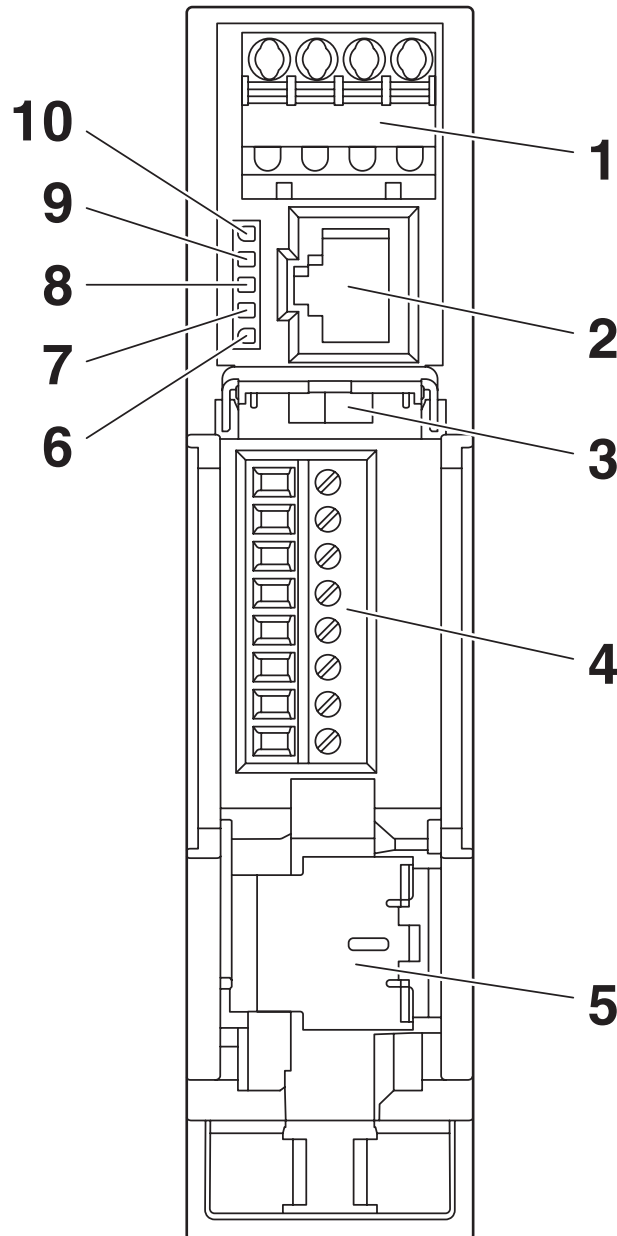
Schemazeichnung
