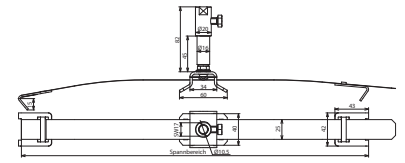
Maßbild HA 10 1F FG120.300 V2A
