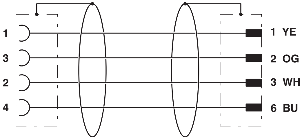
Kontaktbelegung der M12-Buchse und des RJ45-Steckers
