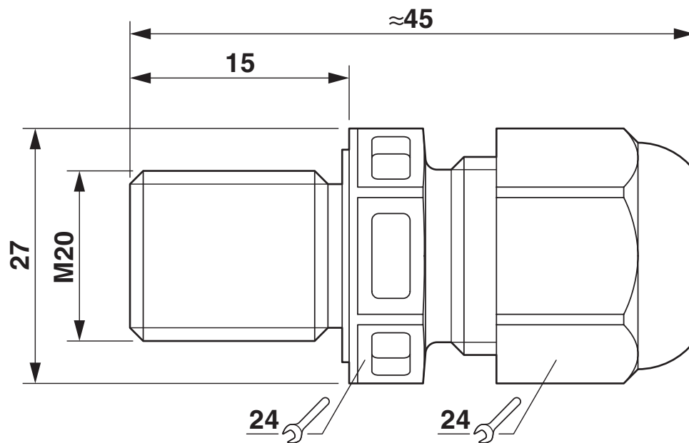
Maßzeichnung
