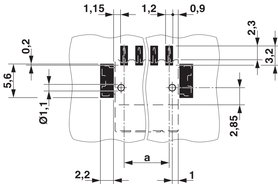
Esquema de taladros/geometría pads soldadura
