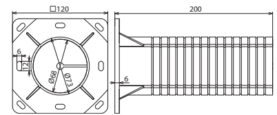
Maßbild AH TSK WDVS 50.200 K
