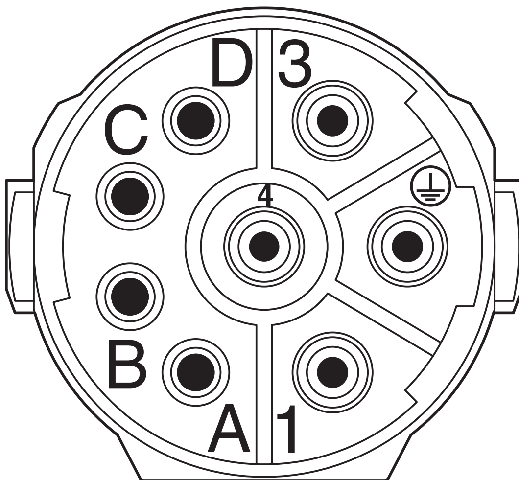
Plano esquemático
