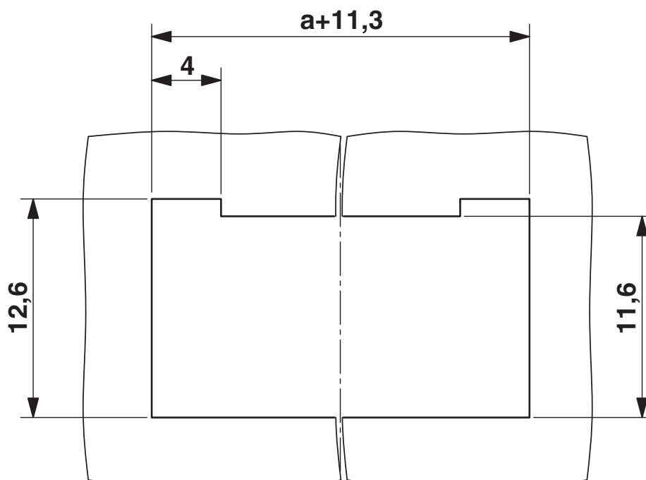
Dessin schématique
