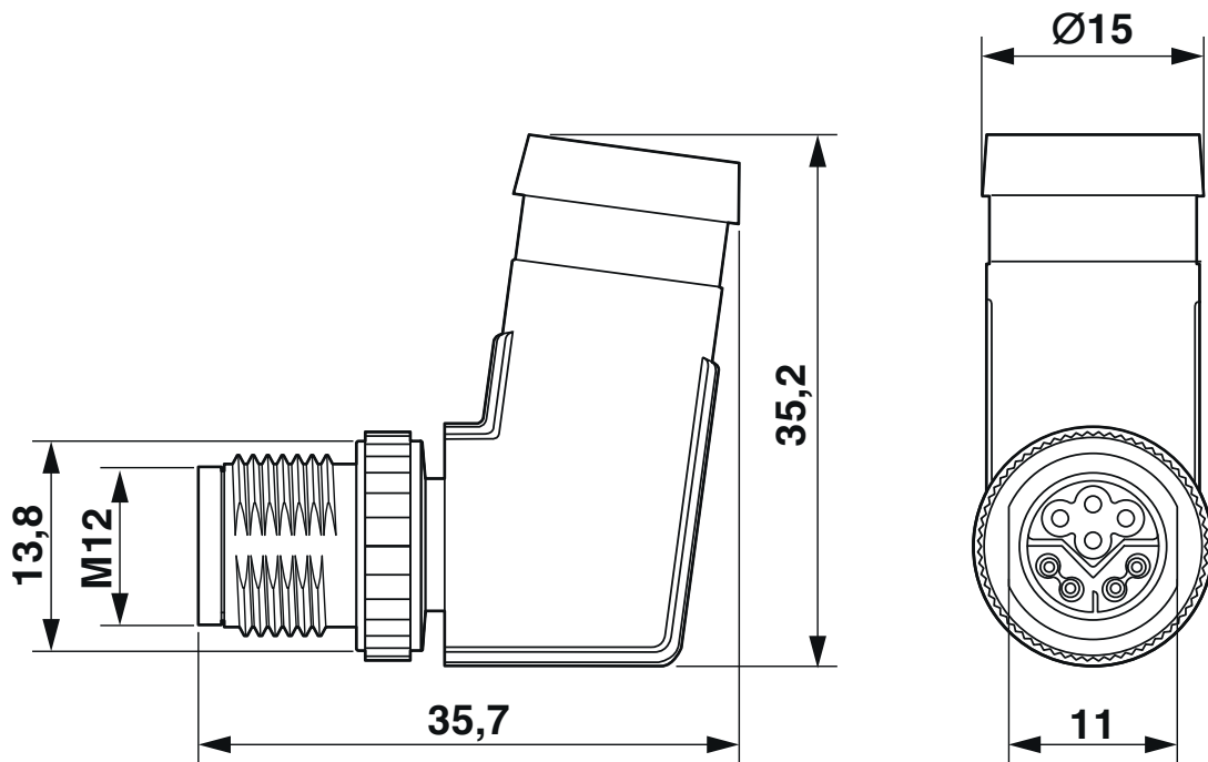
Maßzeichnung
