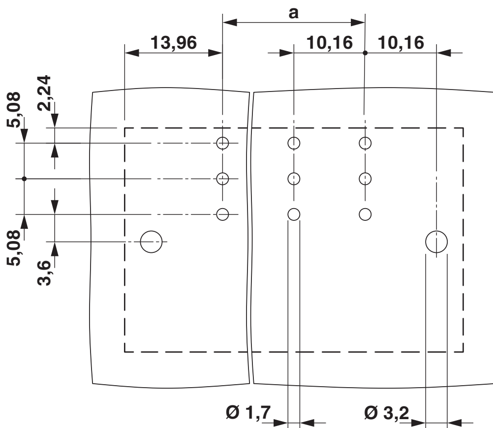
Esquema de taladros/geometría pads soldadura
