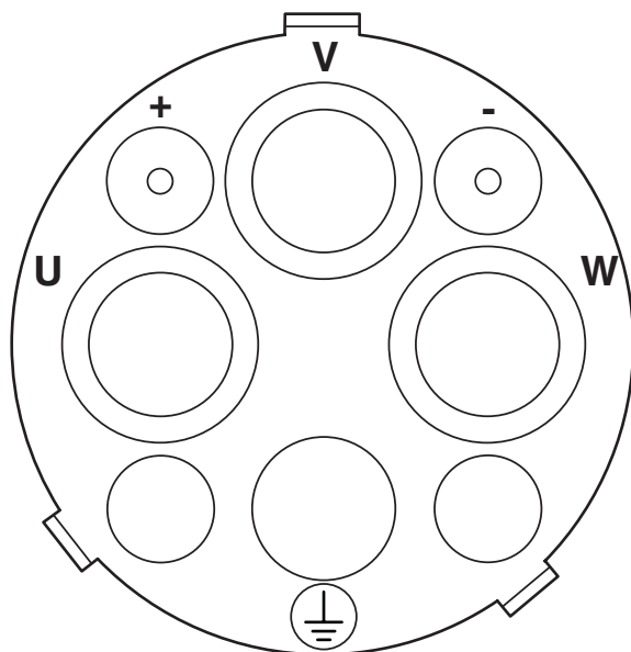
Dessin schématique
