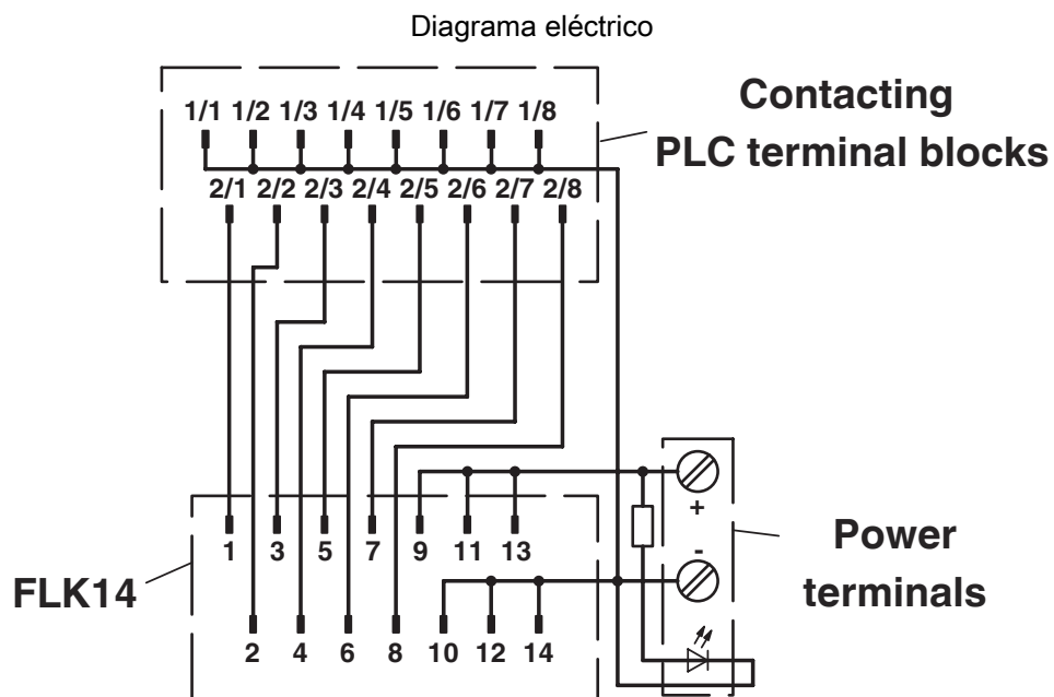
Esquema de conexiones PLC-V8/FLK14/IN/M
