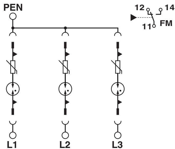
Schaltplan
