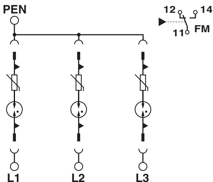
Diagrama eléctrico
