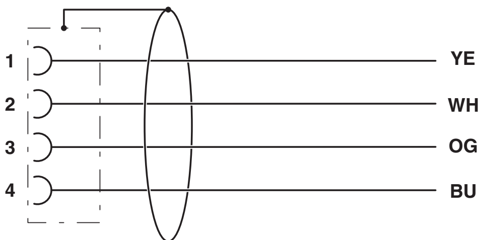
Diagrama eléctrico
