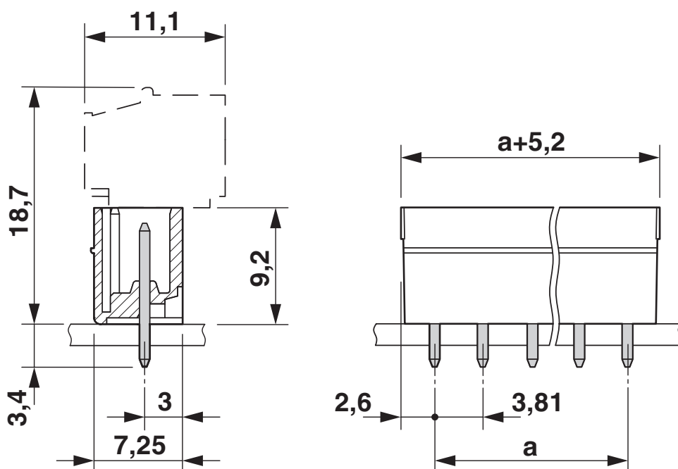
Dessin coté
