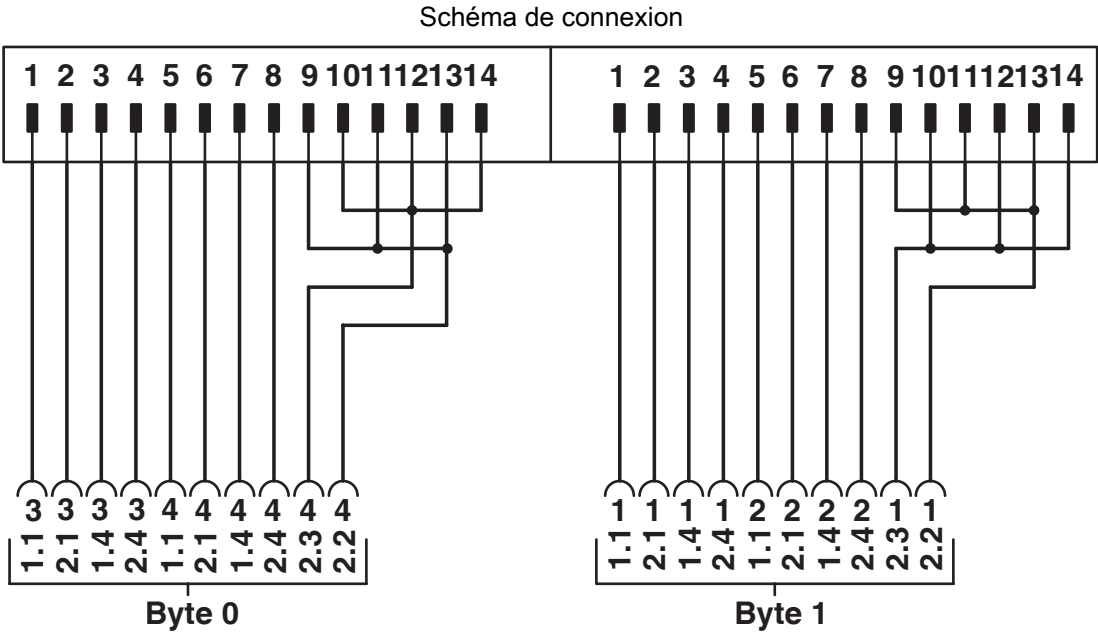
Schéma des connexions FLKM 14-PA-INLINE/IN16
