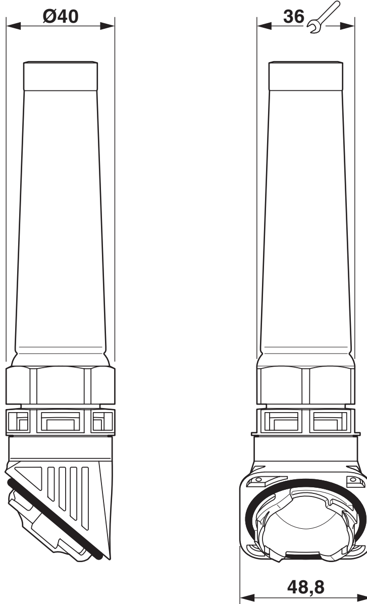
Dessin coté
