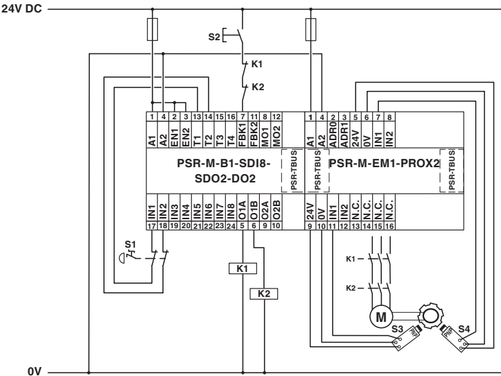
Applikationszeichnung
