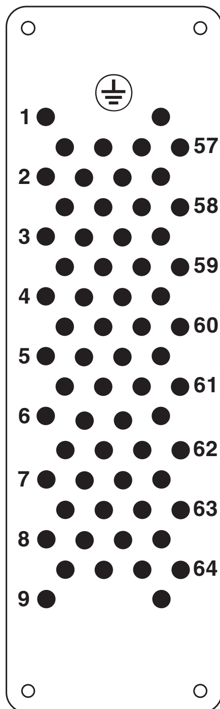
Plano esquemático
