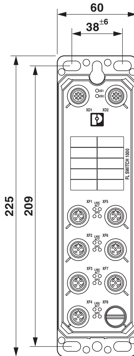
Esquema de dimensiones
