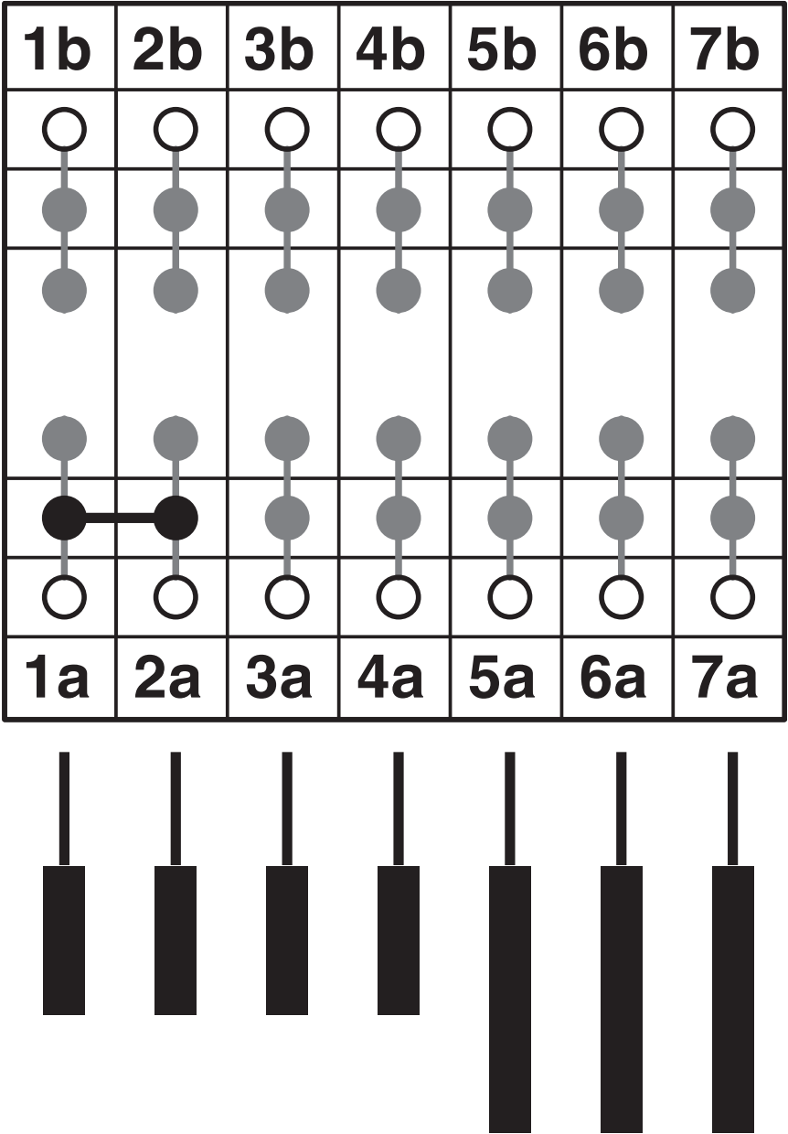
Diagrama eléctrico
