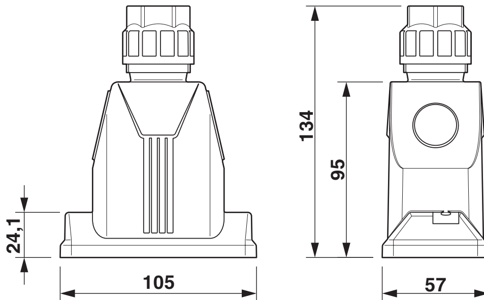
Maßzeichnung
