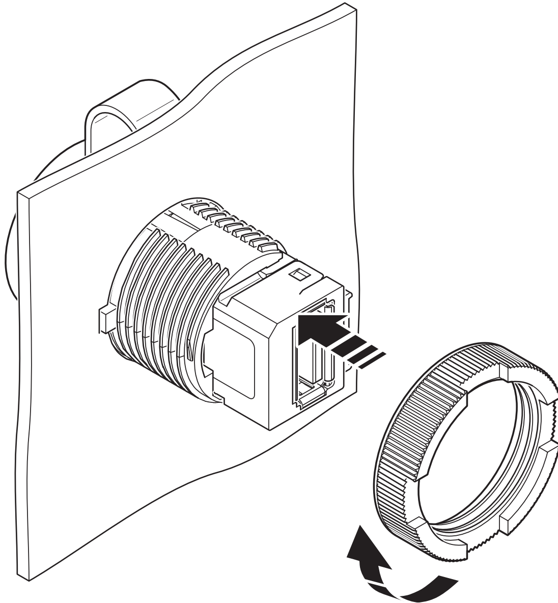
Schemazeichnung
