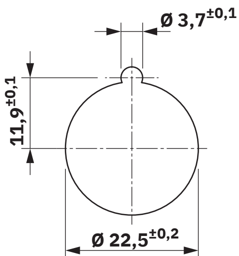
Maßzeichnung
