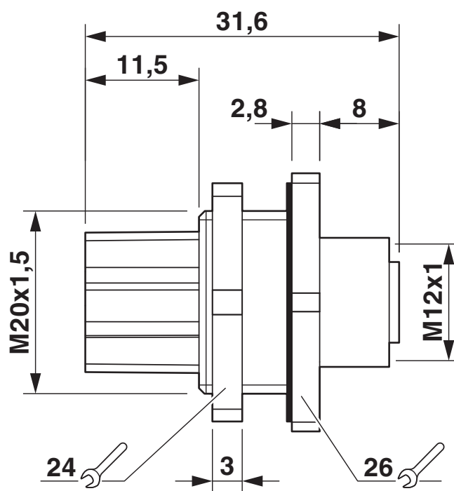
Maßzeichnung
