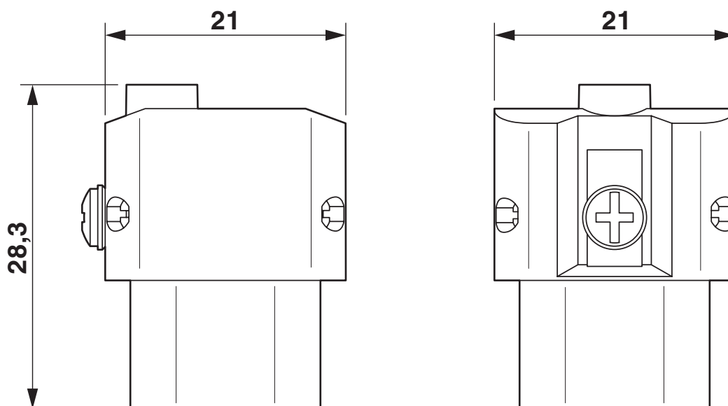
Maßzeichnung
