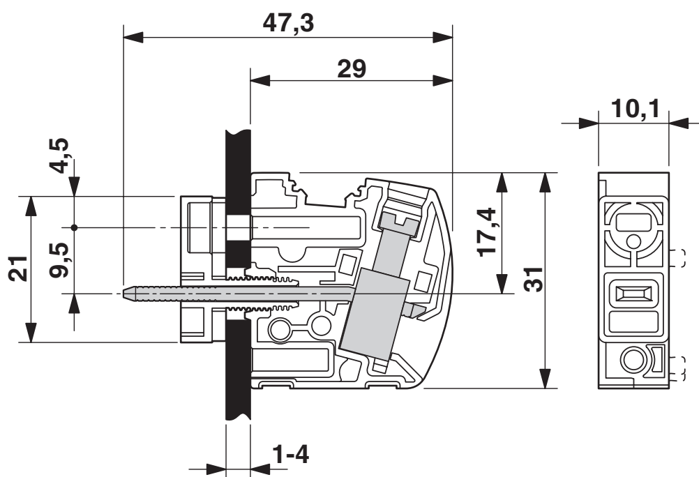
Dessin coté
