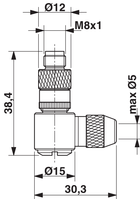
Maßzeichnung
